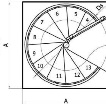
Přídorys
